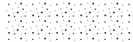
ЗВЁЗДНОЕ НЕБО
