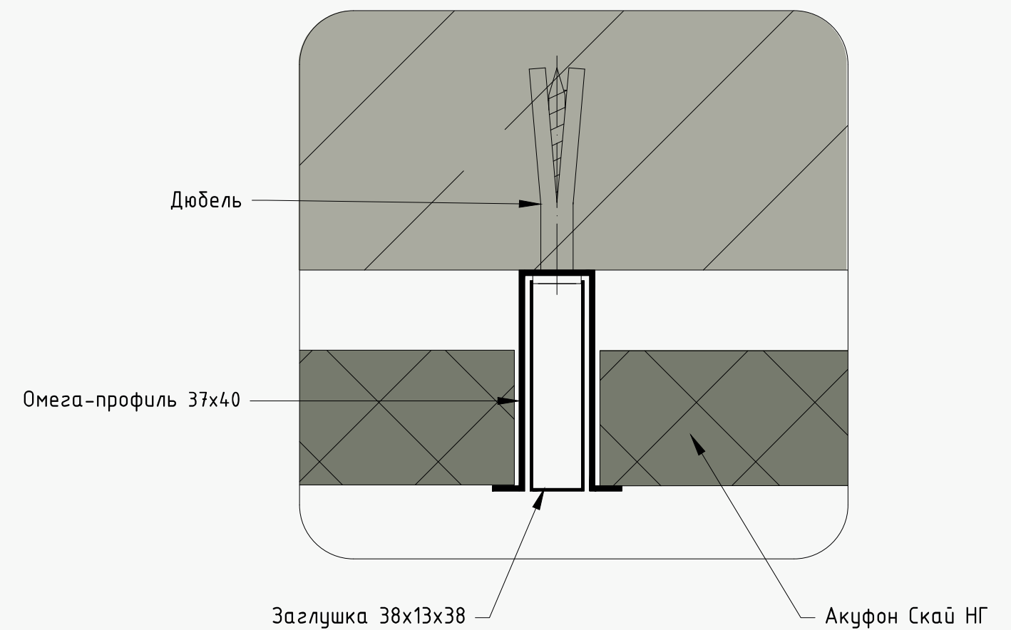
Узел Б
