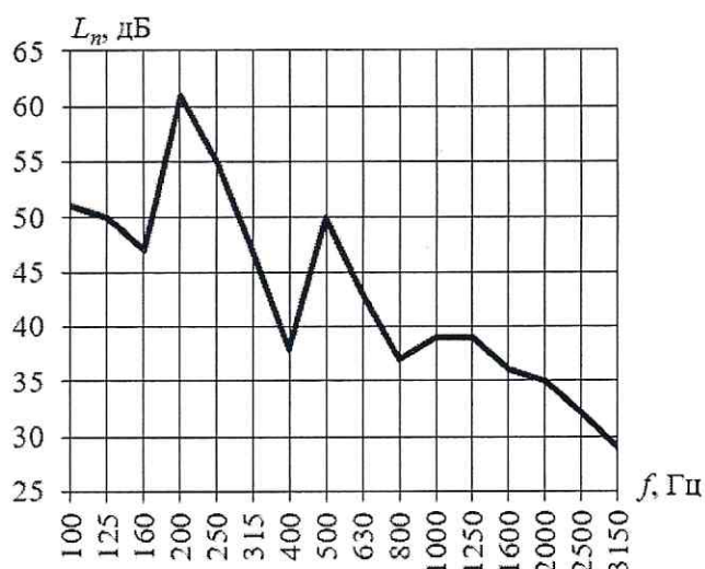
Рисунок - Частотная характеристика приведенного уровня ударного шума под перекрытием с конструкцией пола
