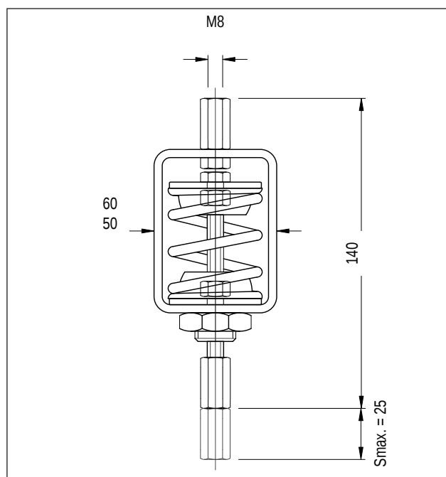
Рисунок ISOTOP® MSN/Z
