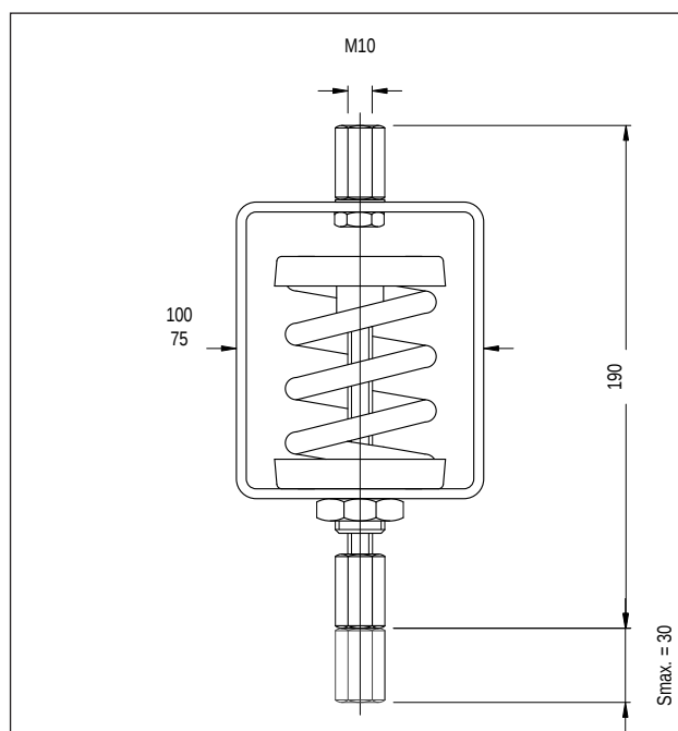
Рисунок ISOTOP® SD/Z
