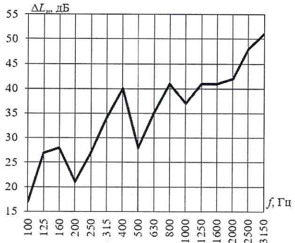
Рисунок - Частотная характеристика улучшения изоляции ударного шума под перекрытием конструкцией пола
