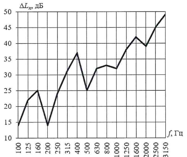
Рисунок - Частотная характеристика улучшения изоляции ударного шума под перекрытием конструкцией пола
