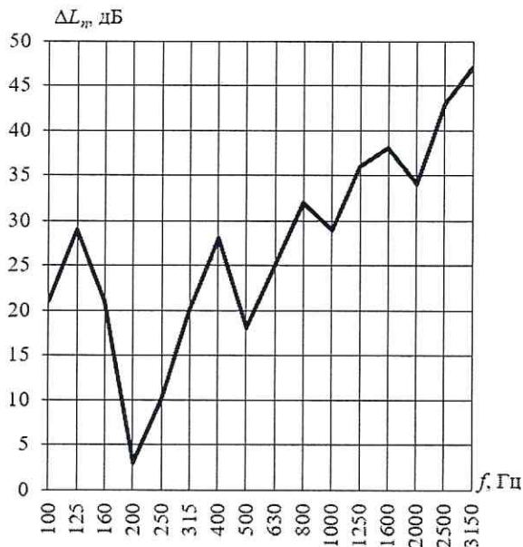
Рисунок - Частотная характеристика улучшения изоляции ударного шума под перекрытием конструкцией пола
