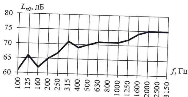
Рисунок - Частотная характеристика приведенного уровня ударного шума под перекрытием без конструкции пола
