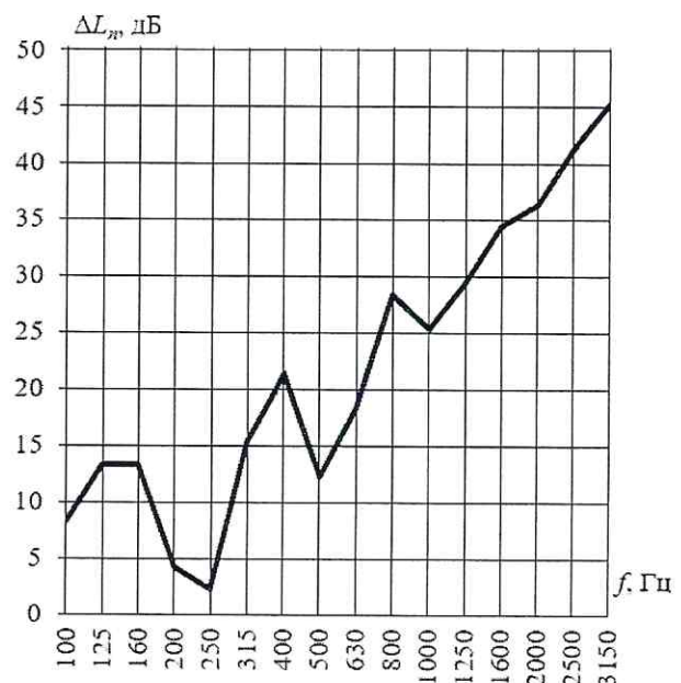
Рисунок - Частотная характеристика улучшения изоляции ударного шума под перекрытием конструкцией пола
