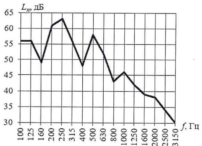
Рисунок - Частотная характеристика приведенного уровня ударного шума под перекрытием с конструкцией пола
