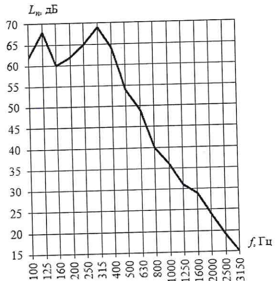
Рисунок - Частотная характеристика приведенного уровня ударного шума под перекрытием с конструкцией пола
