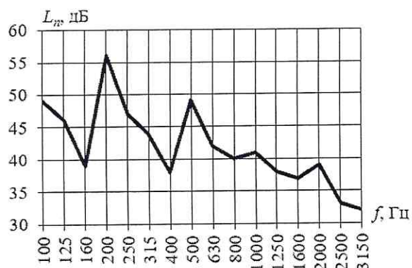
Рисунок - Частотная характеристика приведенного уровня ударного шума под перекрытием с конструкцией пола
