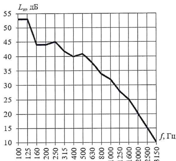
Рисунок - Частотная характеристика приведенного уровня ударного шума под перекрытием с конструкцией пола
