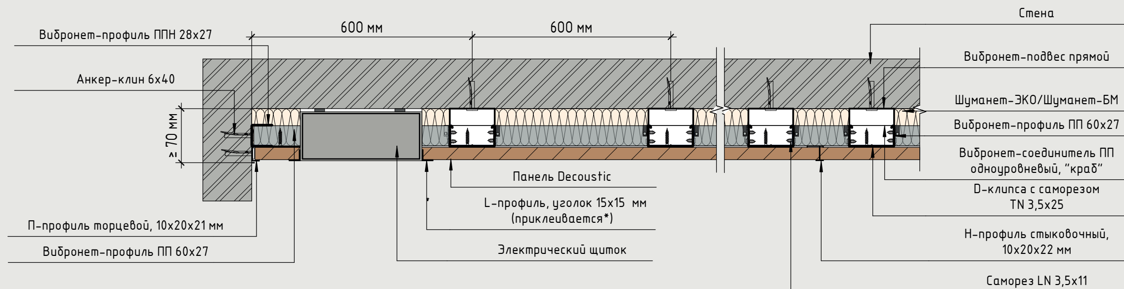
Разрез 14 - 14
