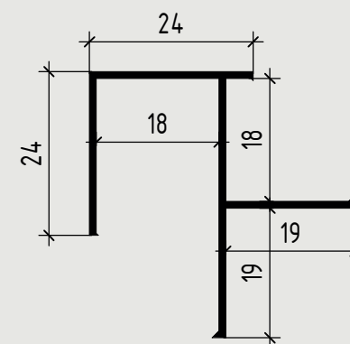
П-профиль установочный
