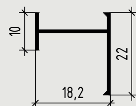
H-профиль стыковочный
