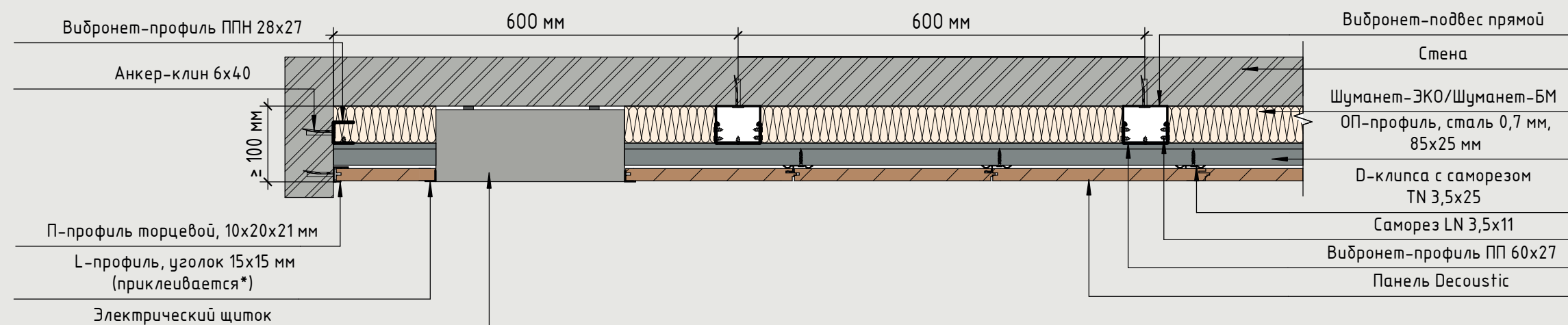
Разрез 7 - 7
