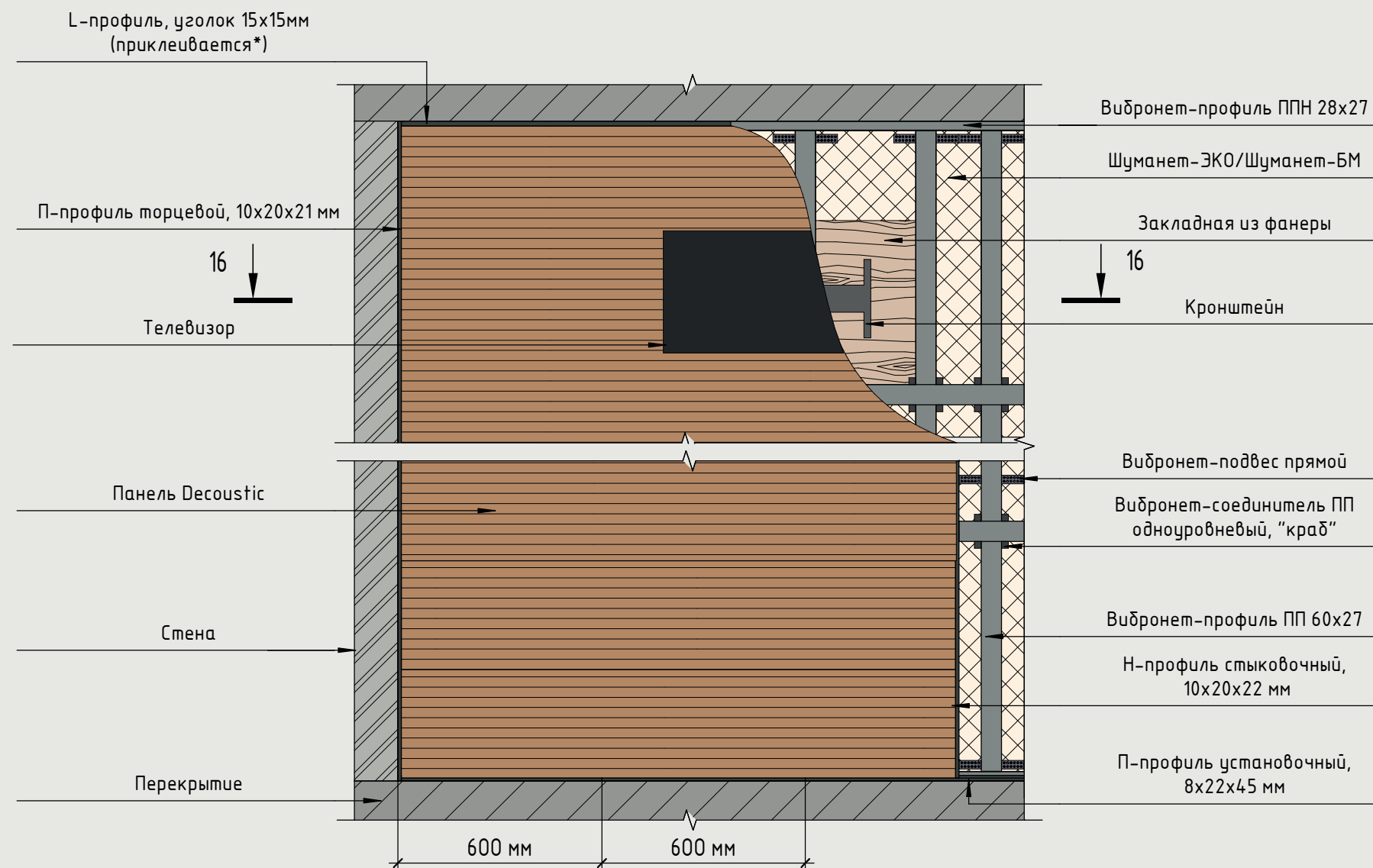
Разрез 16 - 16
