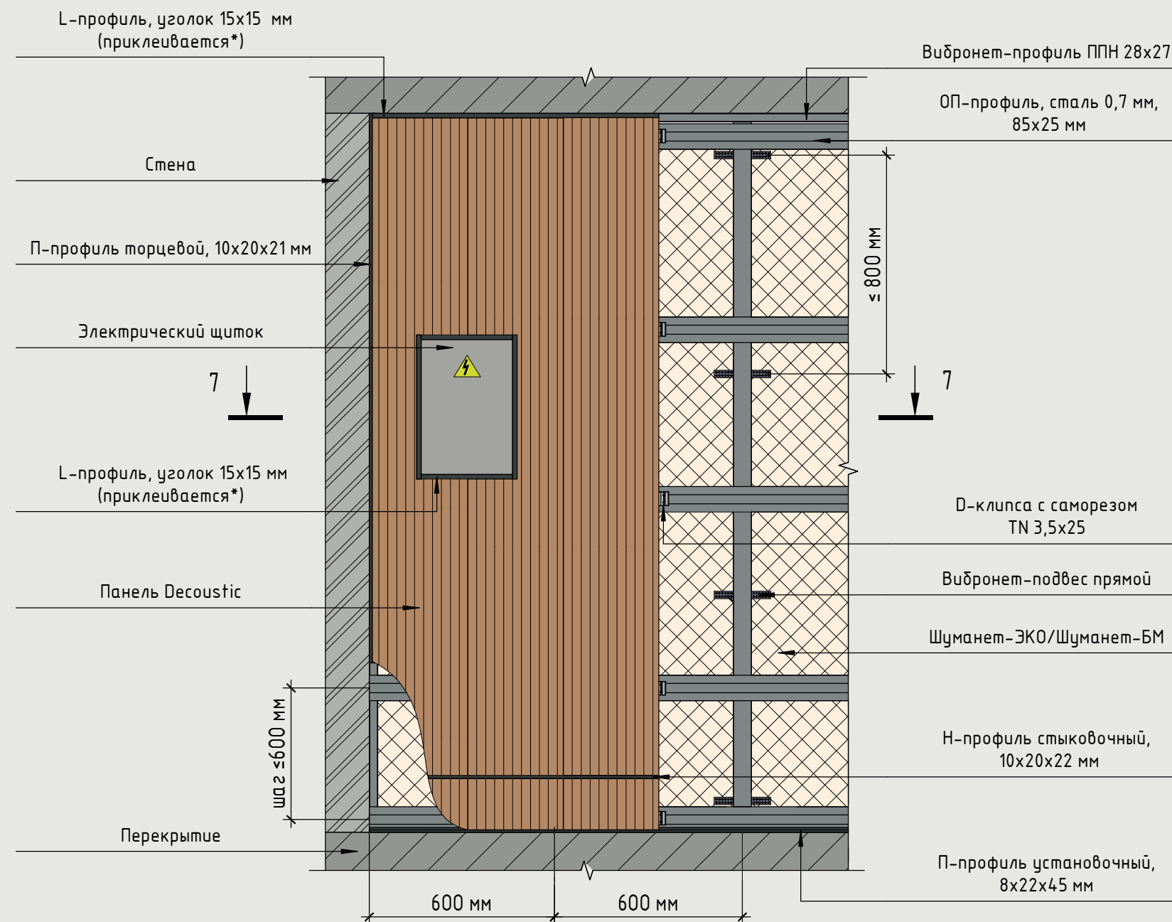
Разрез 7 - 7
