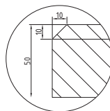
Кромка К10
