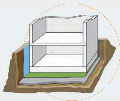
Полноплоскостная опора
