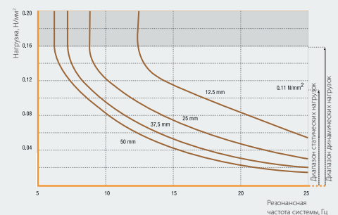
Пример зависимости собственной частоты от нагрузки для материала Sylomer SR110
