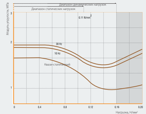
Пример зависимости модуля упругости от нагрузки для материала Sylomer SR110
