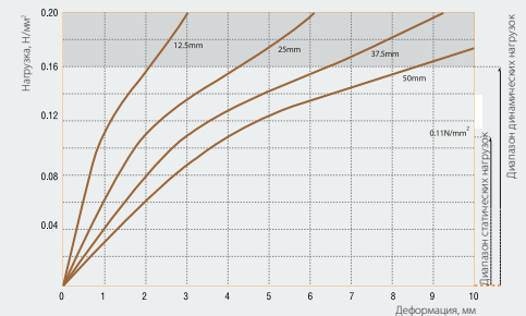
Пример зависимости нагрузки от деформации для материала Sylomer SR110
