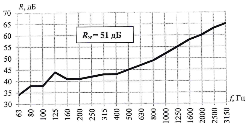
Частотная характеристика звукоизоляции
