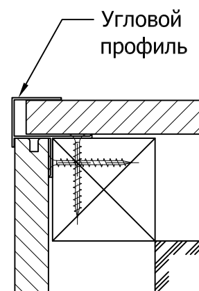
Узел 10 Внешний угол 90°
