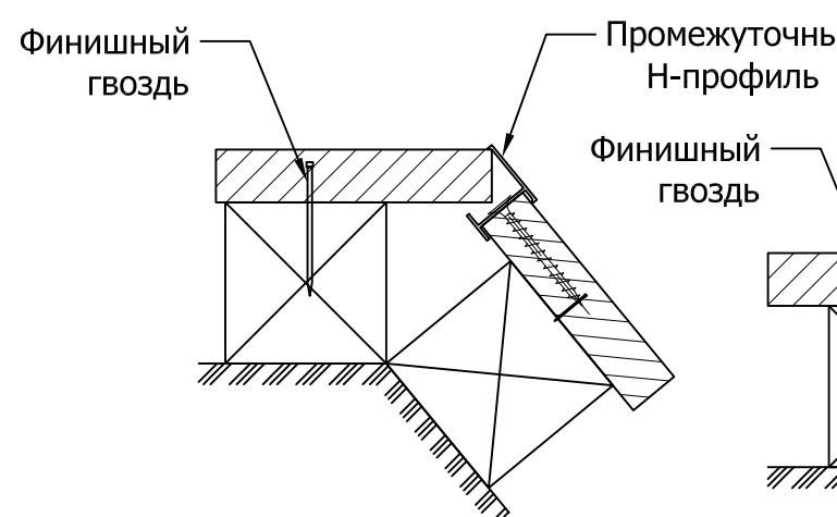
Узел 11 Внешний угол
